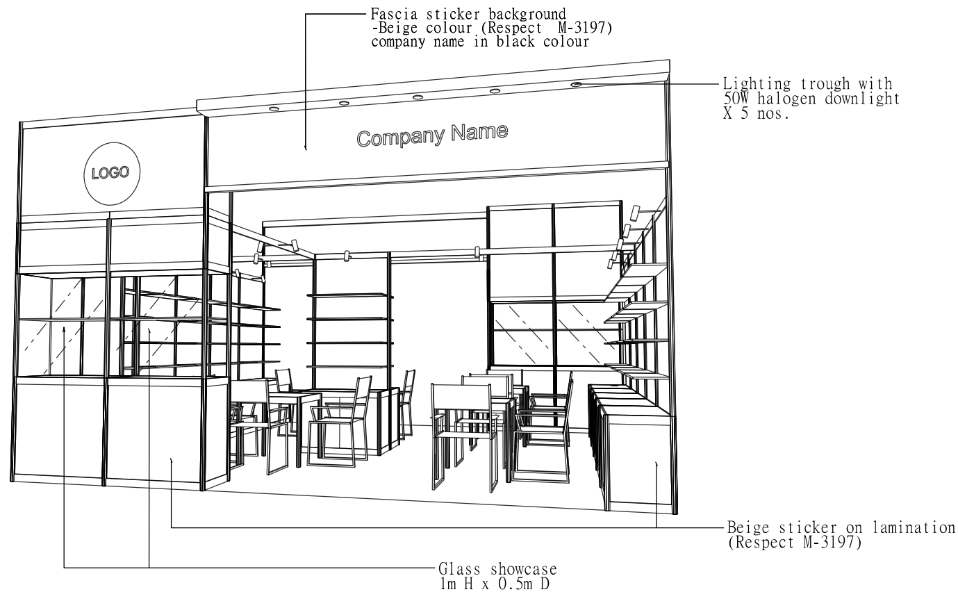
PERSPECTIVE N.T.S
