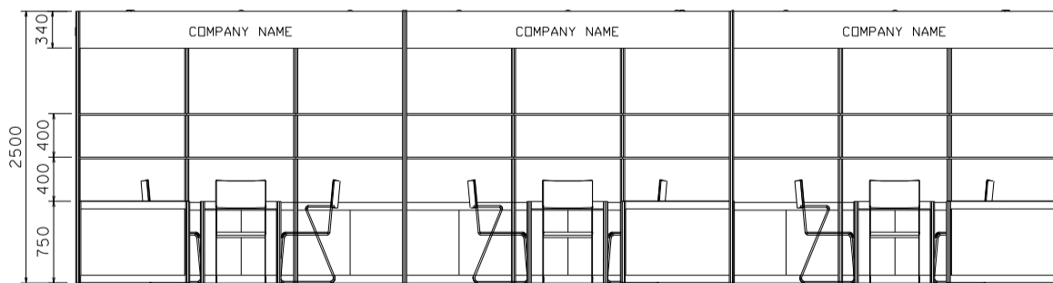
ELEVATION
