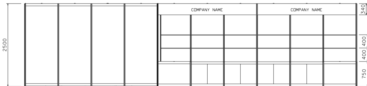
ELEVATION
