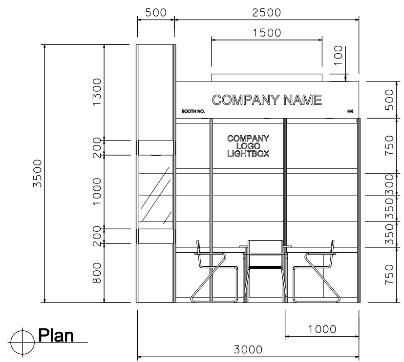
Top Elevation
