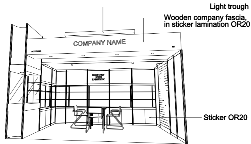
PERSPECTIVE N.T.S
